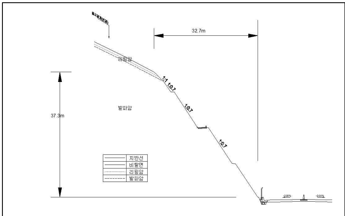
【대표단면 Sta.3+330~3+520(상주)】
