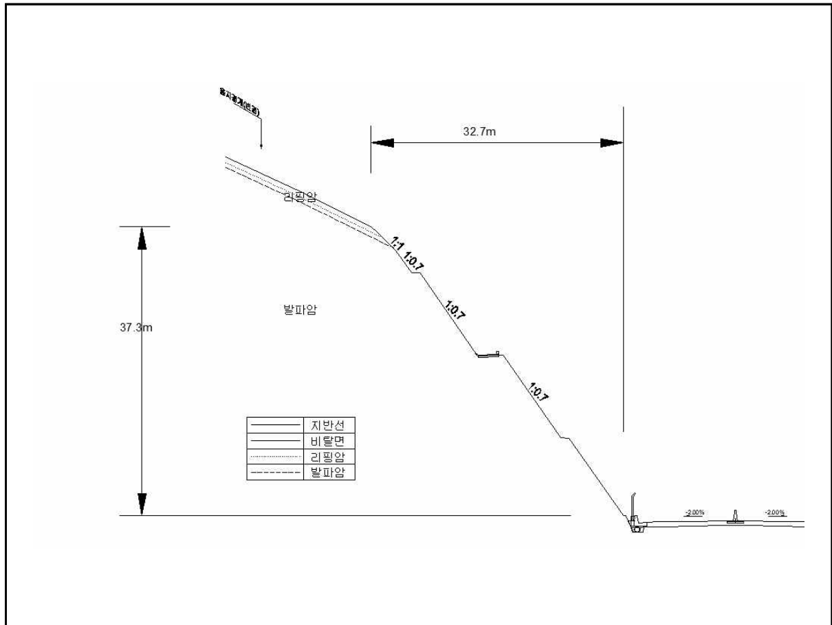
【대표단면 Sta.3+380(상주)】
