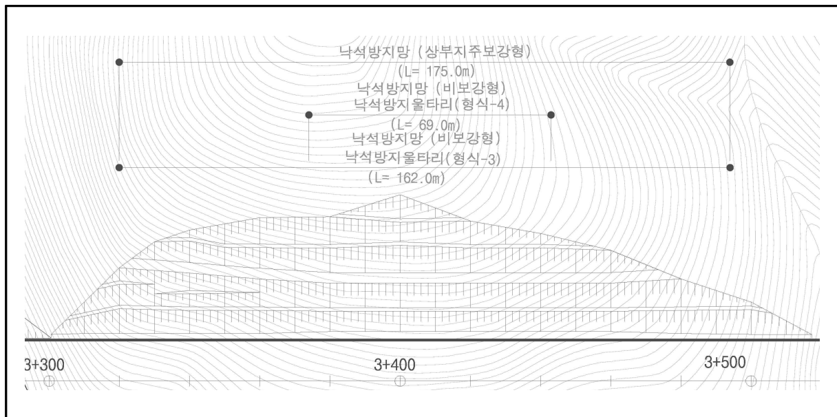
【Sta.3+330~3+520(상주)】
